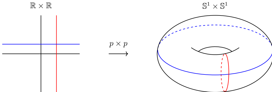
Figura 1.10: Ejemplo de recubridor del toro.
